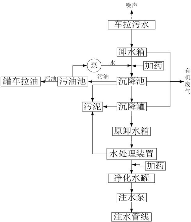
图 2-1 项目运营期生产工艺及产污环节图
