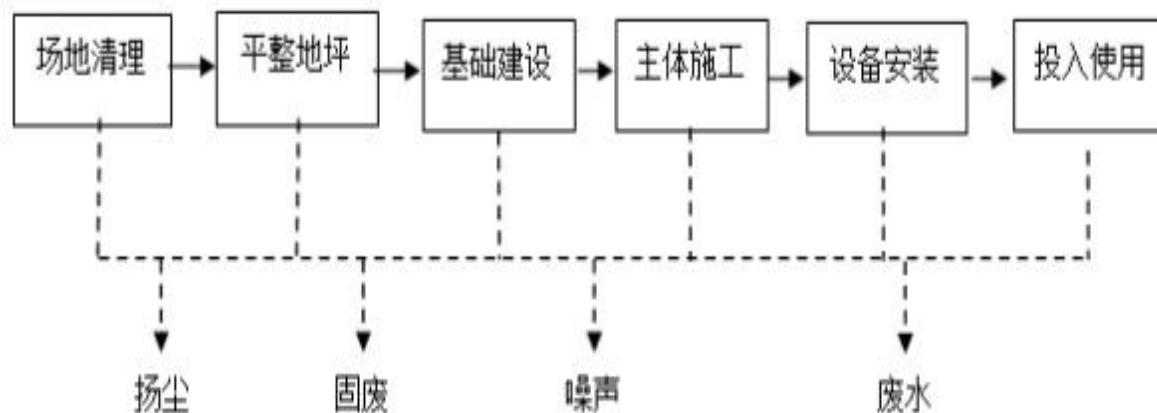
图2-1 站场施工建设工艺流程及产污环节图
