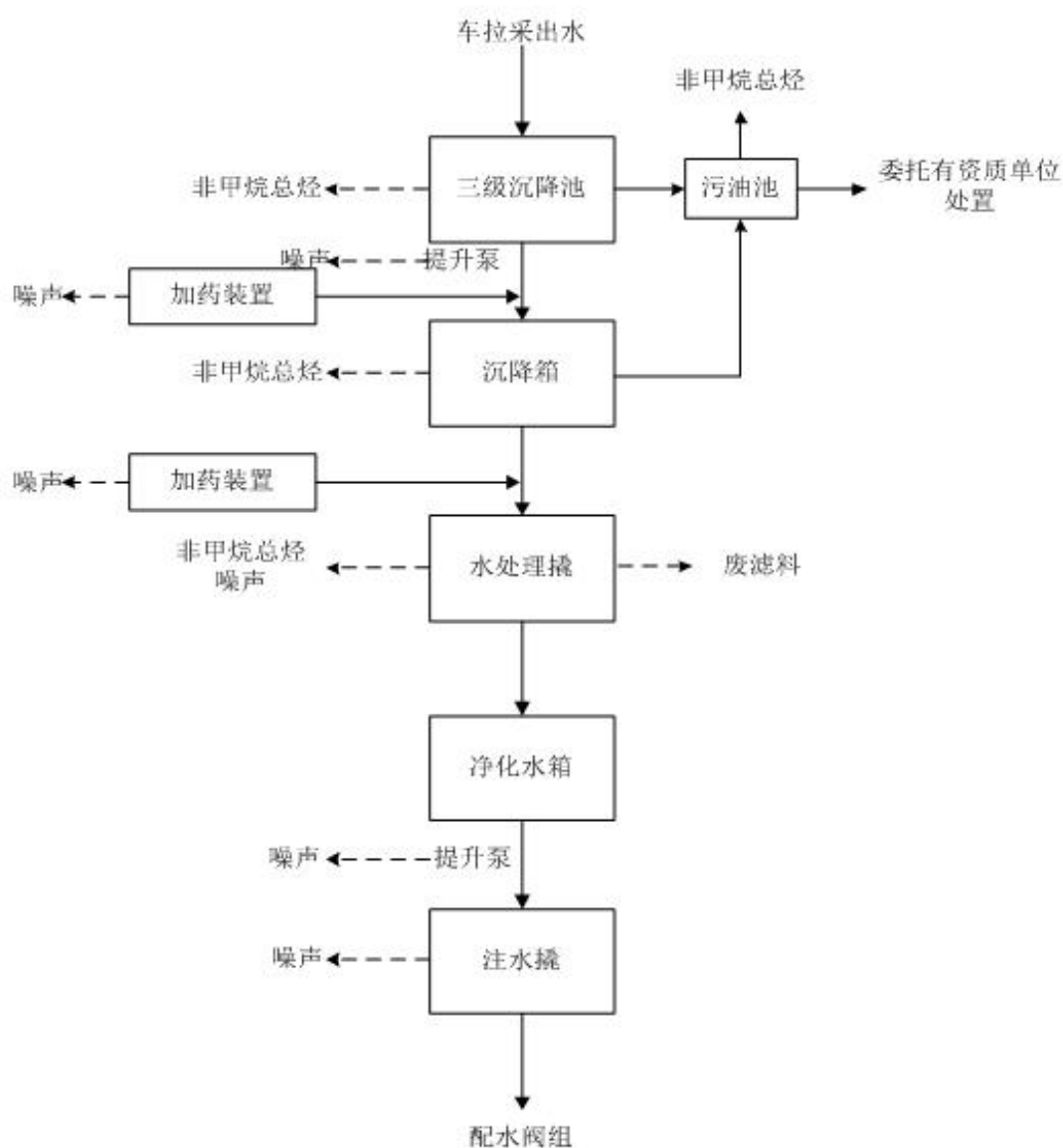
图 2-5 项目工艺流程图
