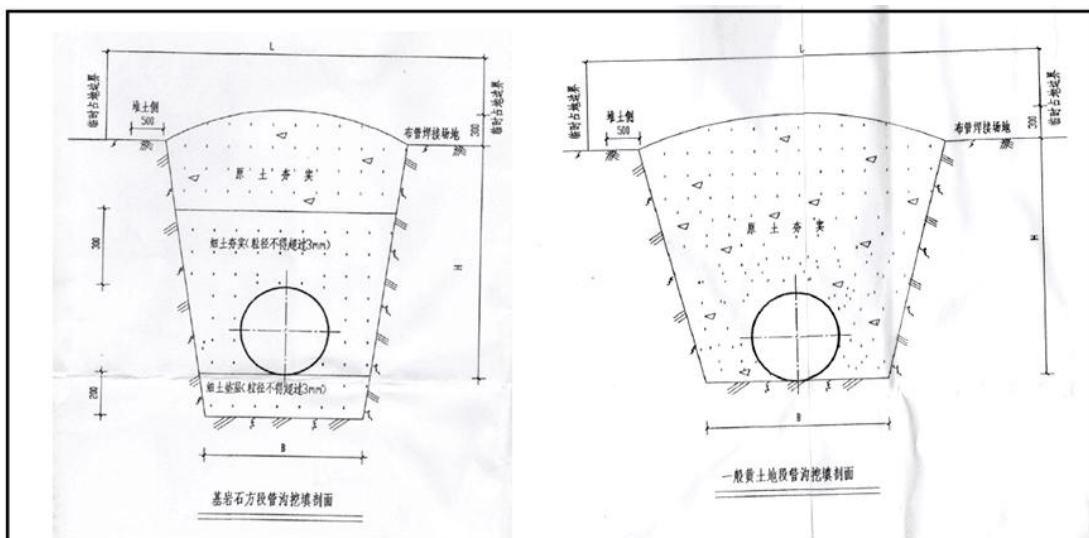
图2-3 管线施工剖面图
