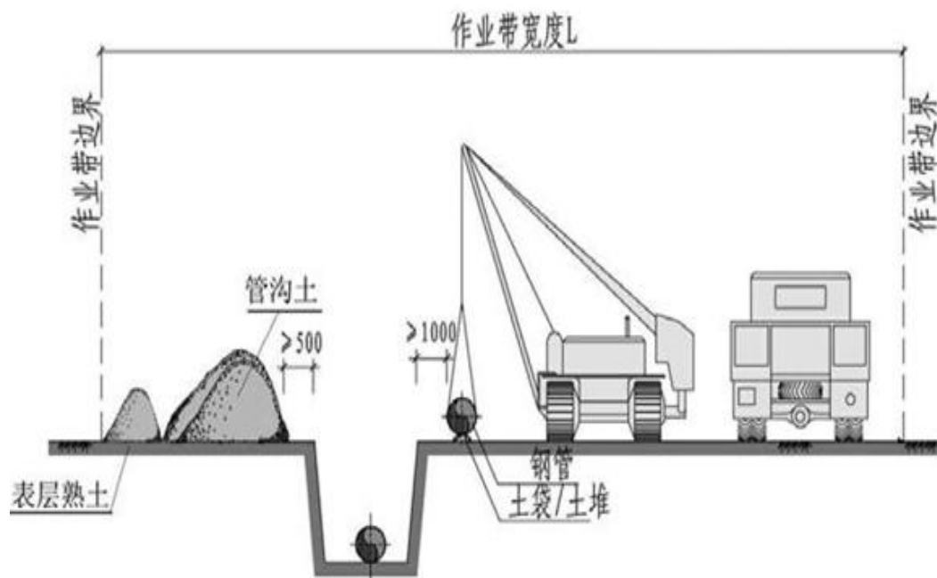
图2-4 管道大开挖施工工艺示意图
