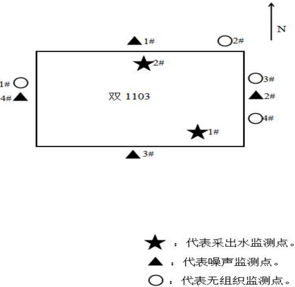
图 5-1 验收监测点位布设示意图
