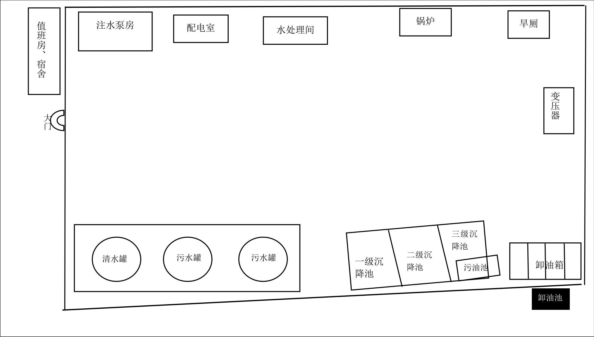
附件 3：厂区平面布置图
