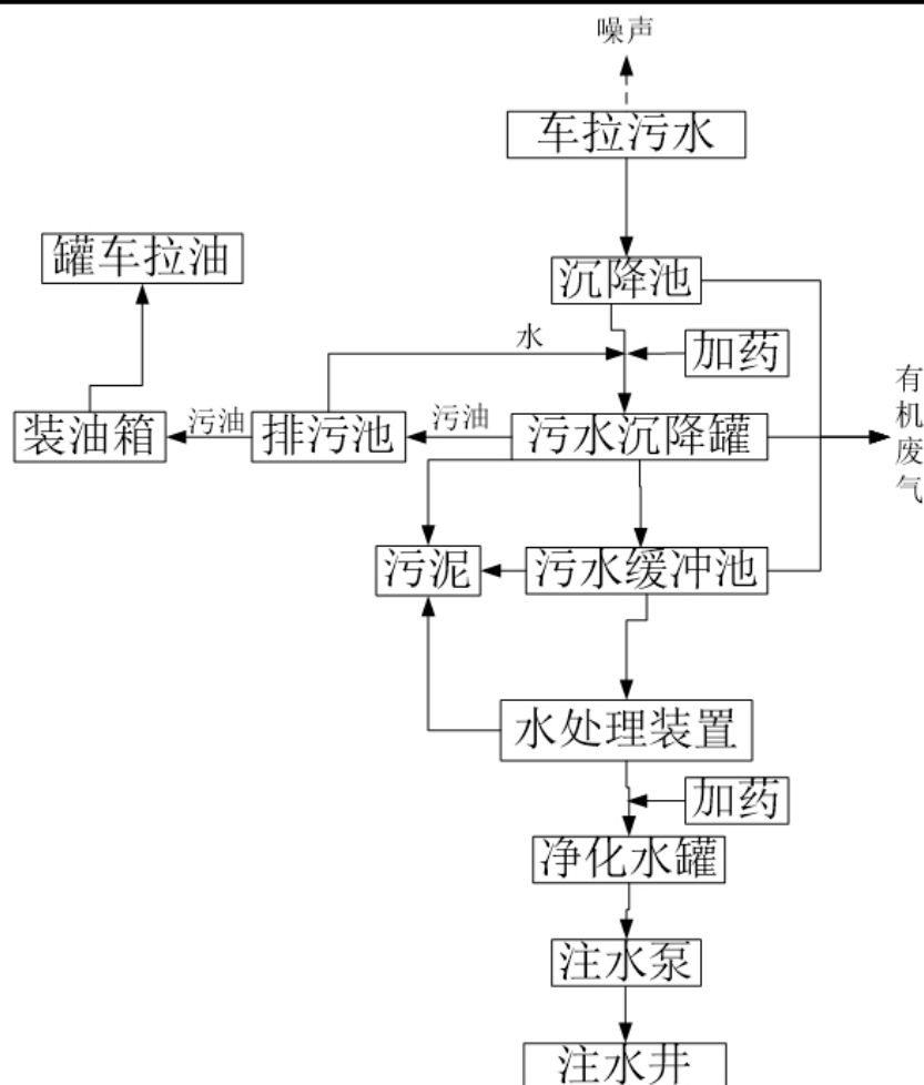
图 3-1 工艺流程图及产污环节
