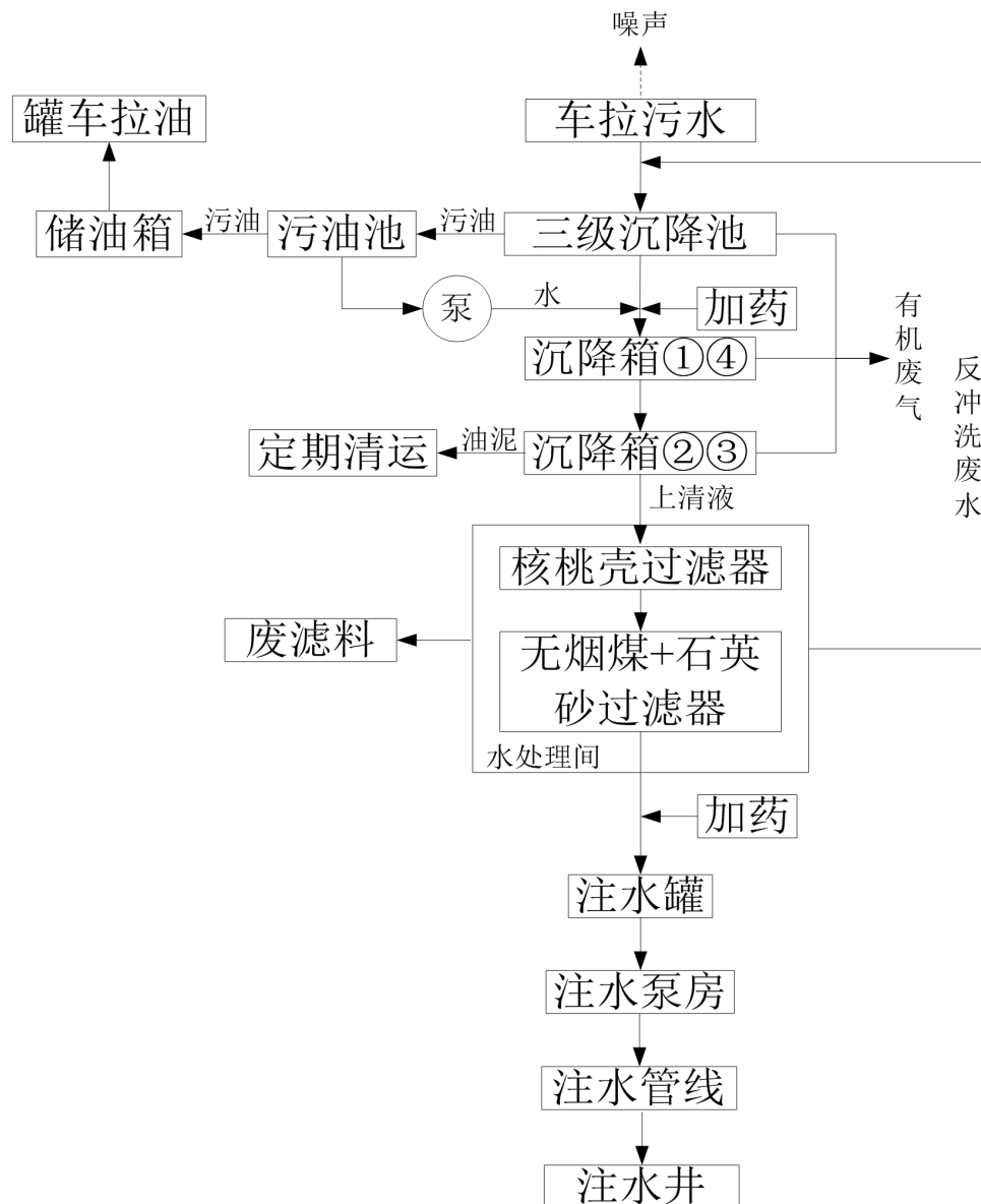
图 3-1 工艺流程图及产污环节
