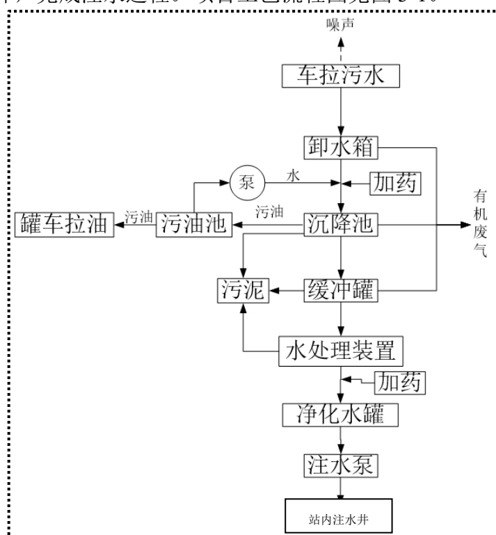
图 3-1 项目工艺流程图
